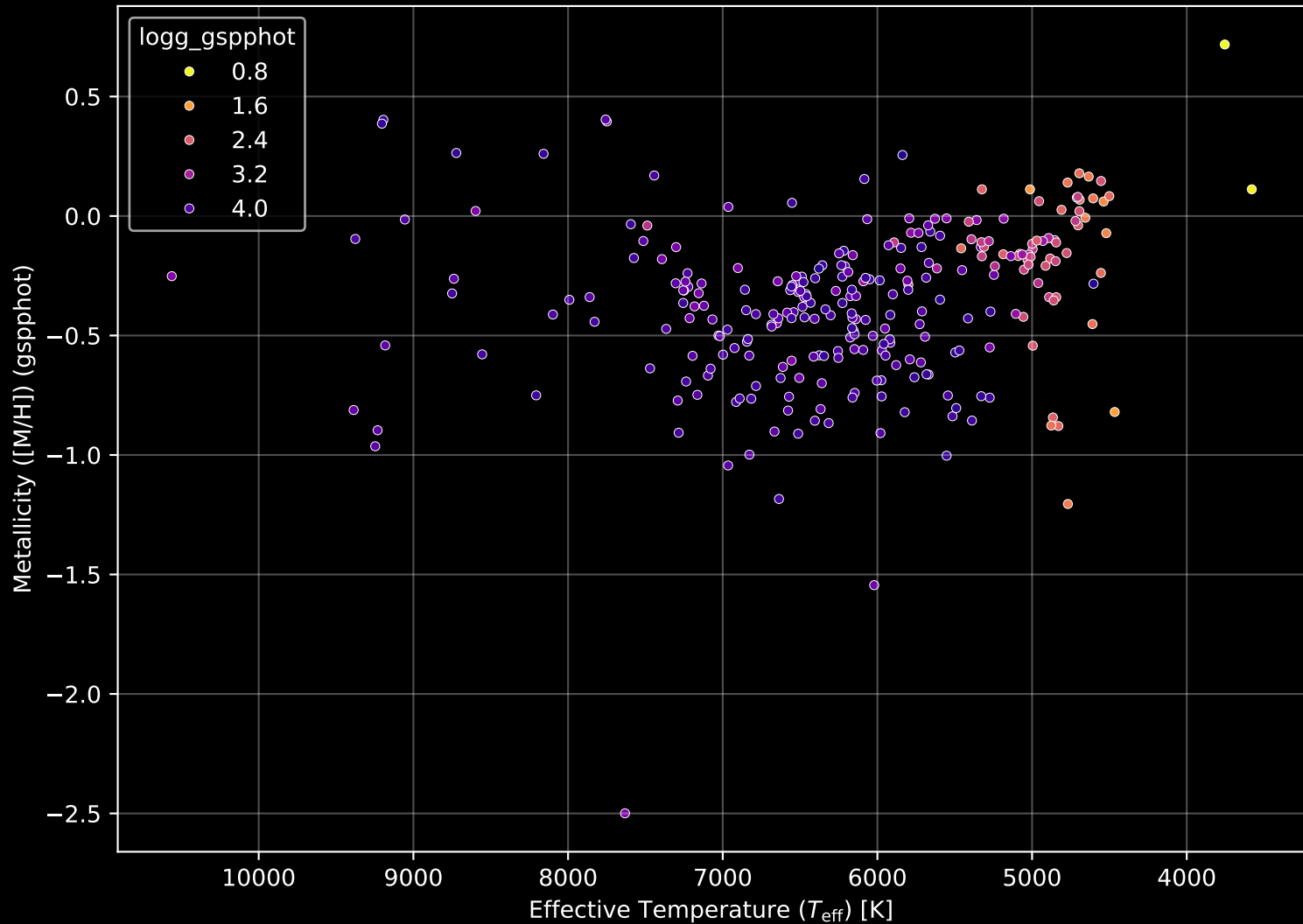
GALAH DR4 Field: [8753] Stellar Population Parameters (n= 277)
