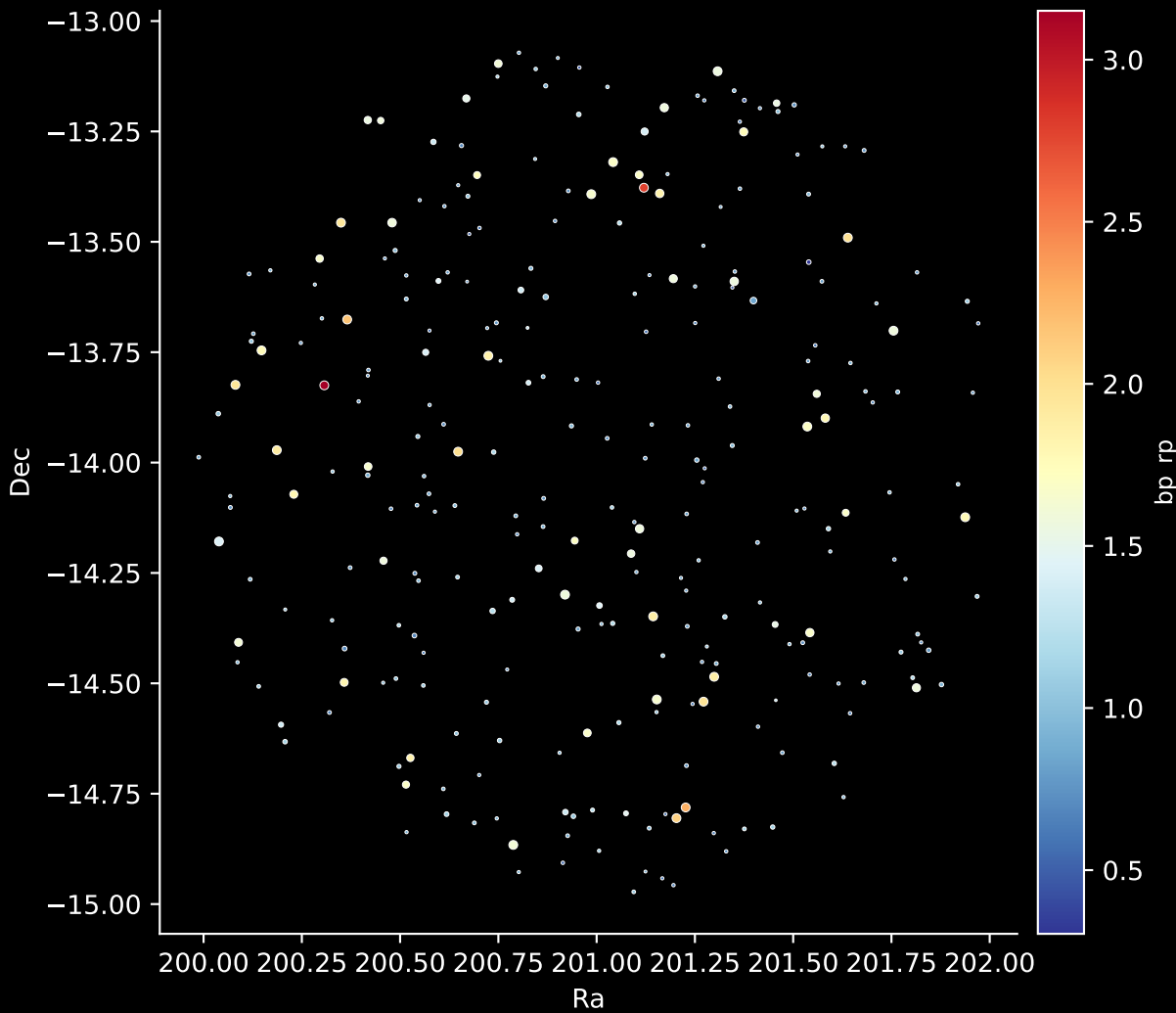
GALAH DR4 Field: [8753] Stars: 277
