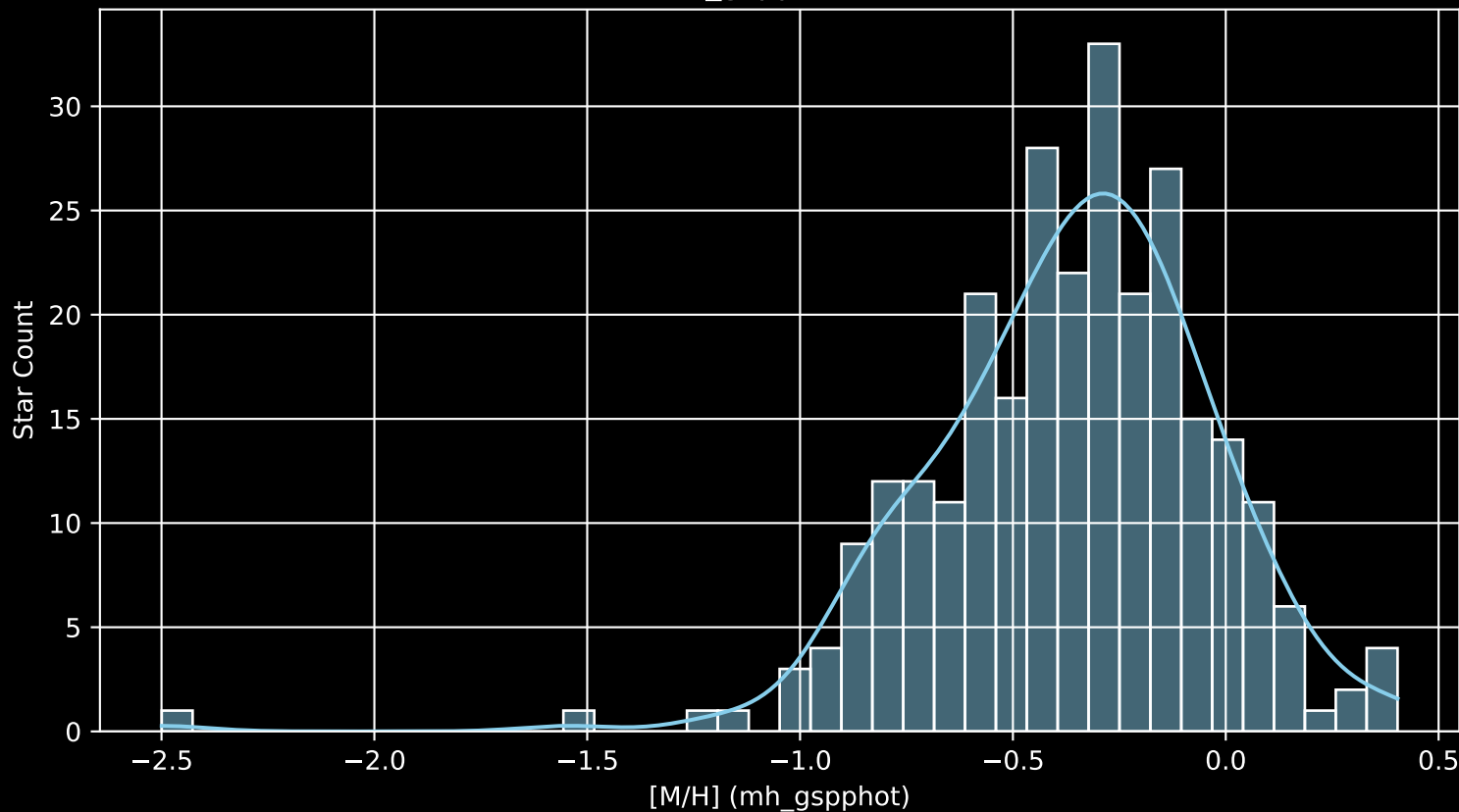
GALAH DR4 Field: [8753] [M/H] (mh_gspphot) (n= 276)
